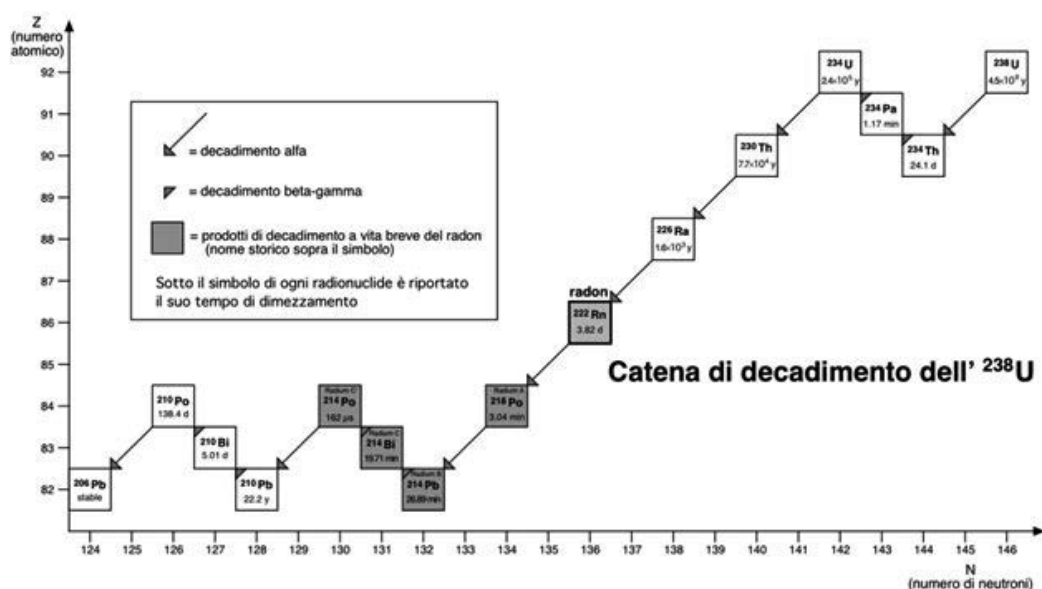
Figura 1: Schema della catena di decadimento dell' ^{238}\text{Uranio} [2]
