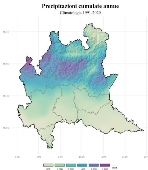
Figura 2.2: Precipitazioni cumulate annue mediate sul periodo climatologico 1991-2020. Dati ArcIS, elaborazione ARPA Lombardia. Sulla geografia della mappa si riportano le Zone omogenee di allerta per il rischio incendi boschivi.
