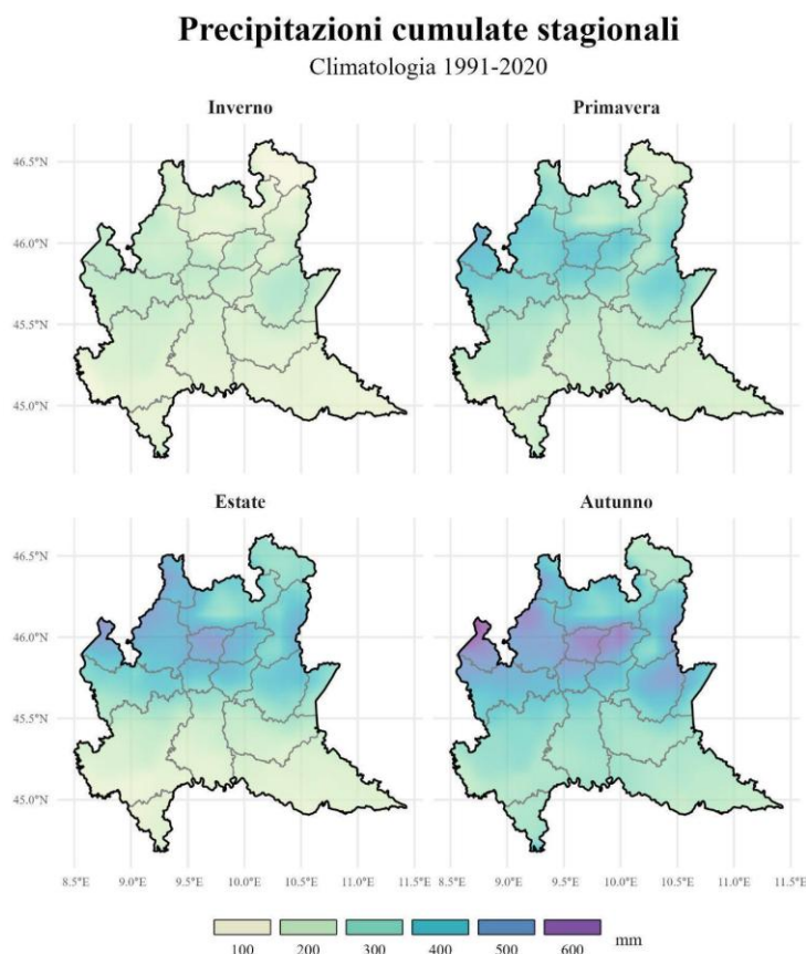
Figura 2.3: Precipitazioni cumulate stagionali mediate sul periodo climatologico 1991-2020. Dati ArCIS, elaborazione ARPA Lombardia.
