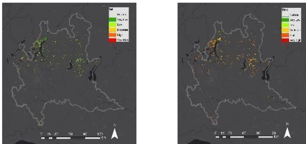
Figura 5.1: classi di pericolosità di FWI (sx) e FFMCI (codice di umidità dei combustibili fini, dx) per gli incendi nel periodo 2002-2018. A causa dell'umidità relativamente elevata dell'area di studio, gli indici a lungo termine come il FWI non spiegano bene il verificarsi di incendi, mentre l'indice a breve termine FFMCI cattura maggiormente la variabilità del fenomeno
