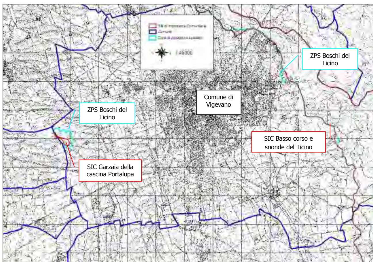
Fig. 3.14 – SIC (in colore rosso) e ZPS (in colore azzurro) facenti parte la Rete Natura 2000 e limitrofi al SIC IT2080013 "Garzaia della Cascina Portalupa".
