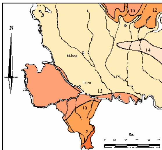
Fig. 3.3 – Stralcio della carta delle temperature medie annue vere (Rossetti & Ottone, 1980). Vigevano rientra nell'area caratterizzata dall'isoterma di 10 °C.
