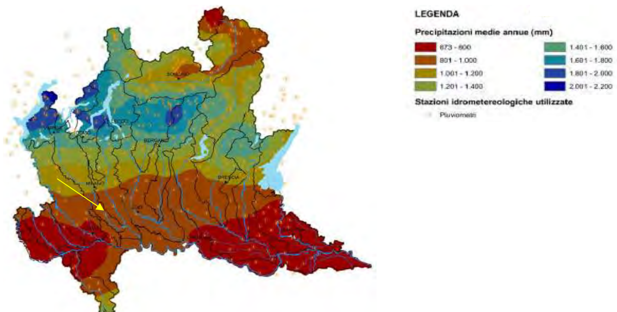
Fig. 3.2 – Stralcio della Carta Regionale delle precipitazioni medie annue con intervallo delle isoiete pari a 200 mm/anno (Regione Lombardia-Direzione Generale Reti e Servizi di Pubblica Utilità, 2004). La freccia gialla indica approssimativamente la posizione del Comune di Vigevano, caratterizzato da precipitazioni comprese tra 600-800 mm/anno.
