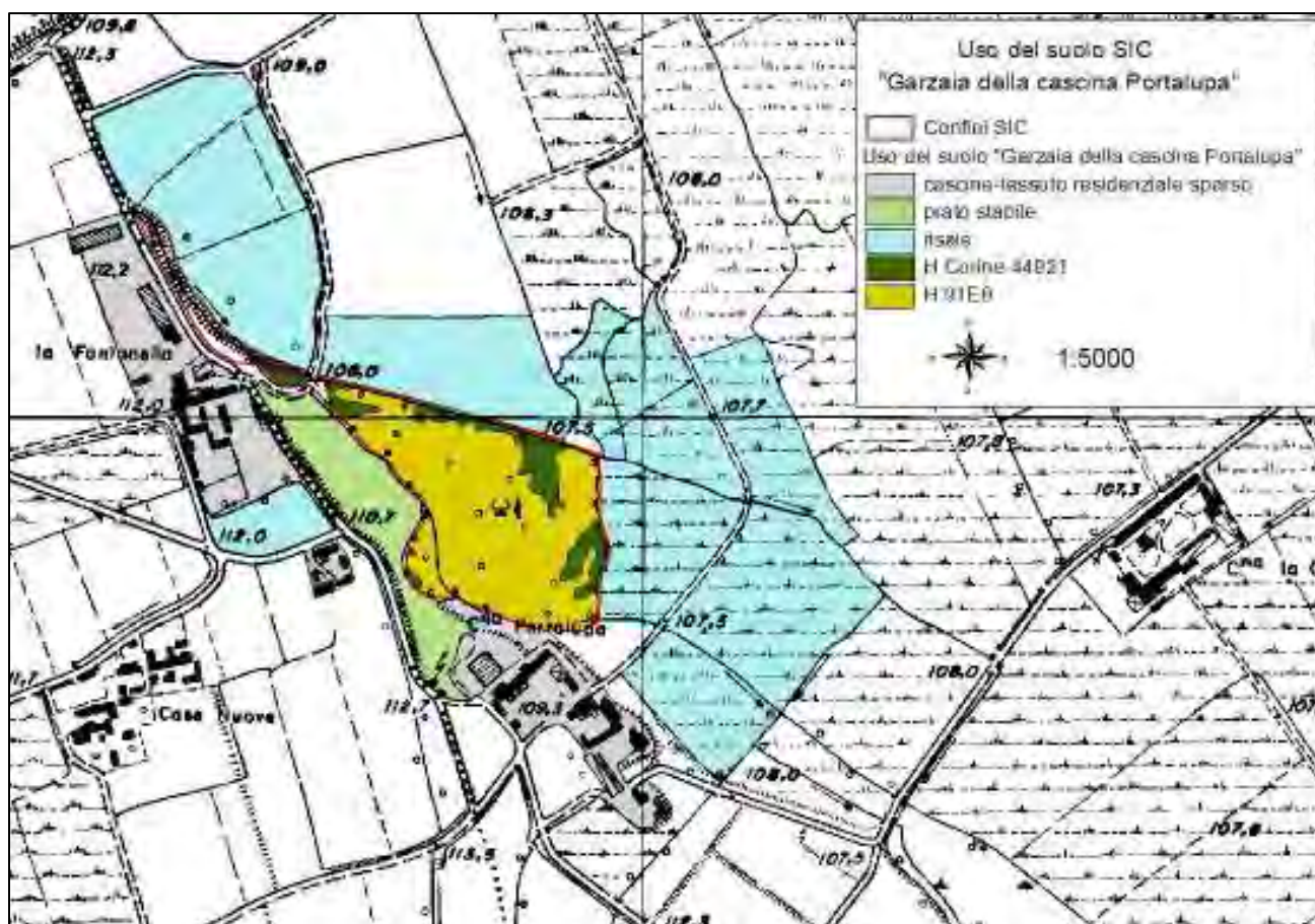
Fig. 3.10 – Restituzione cartografica dell'uso del suolo del SIC "Garzaia della Cascina Portalupa".
