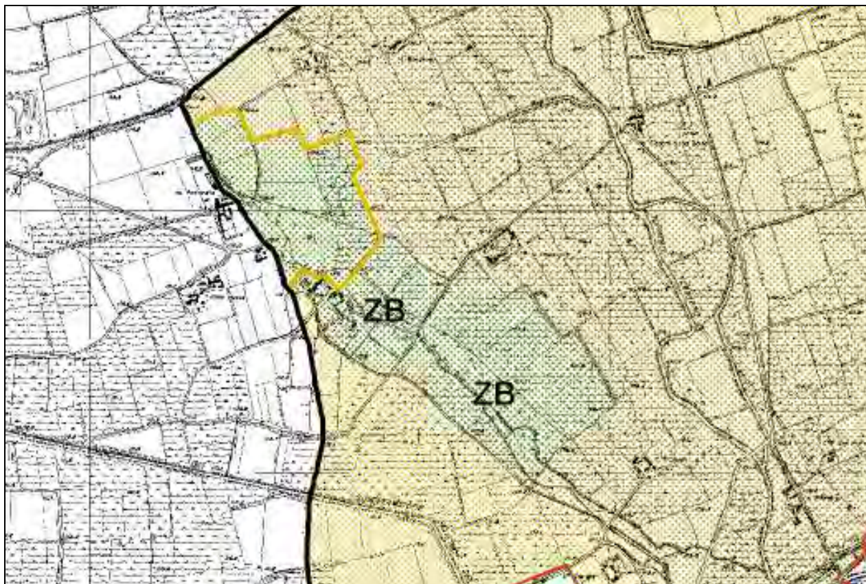
Fig. 3.12 – Estratto dalla cartografia del regime di protezione e dell'azzoneamento del Parco del Ticino e allegata al Piano Territoriale di Coordinamento del Parco stesso. In verde è indicata l'area ZB "Zona naturalistica parziale zoologica-biogenetica".
