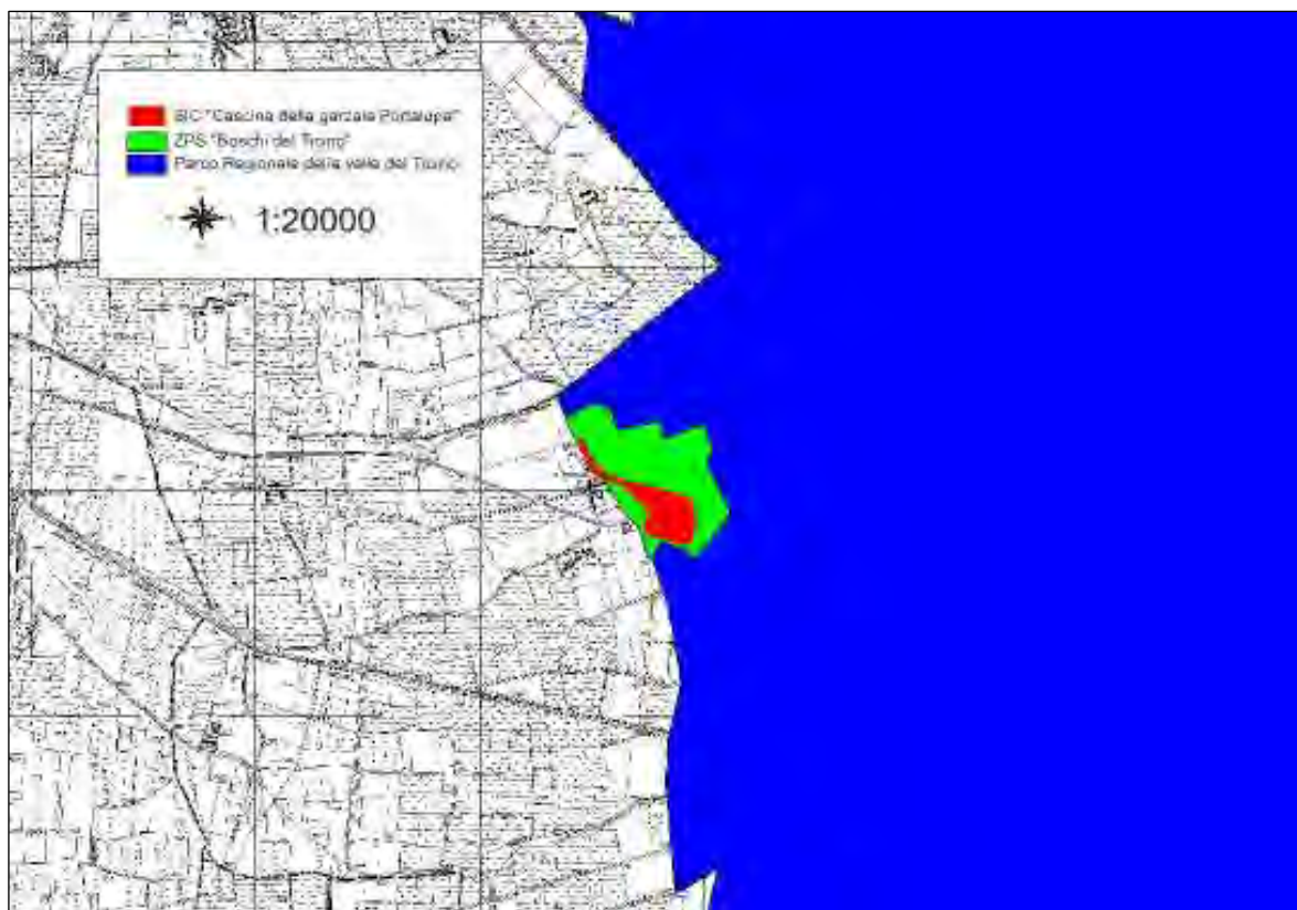
Fig. 3.9 – Il sistema delle aree protette poste nelle vicinanze del SIC "Garzaia della Cascina Portalupa".
