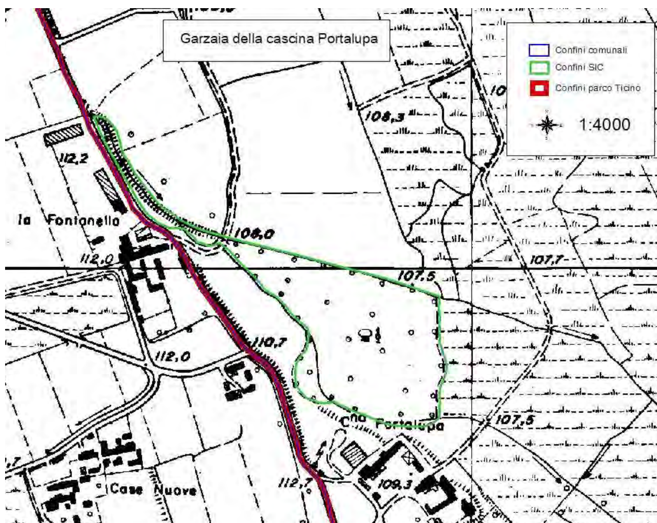
Fig. 3.1 – I confini del SIC "Garzaia della Cascina Portalupa", qui indicati in verde.
