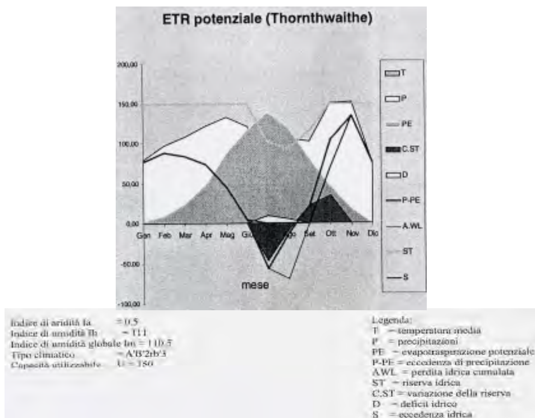
Fig. 3 - Grafico dell'evapotraspirazione potenziale secondo il metodo di Tornhwaite e relativa legenda (Fonte: Piano di Assestamento Forestale Boschi del Turbigaccio 1999-2008).
