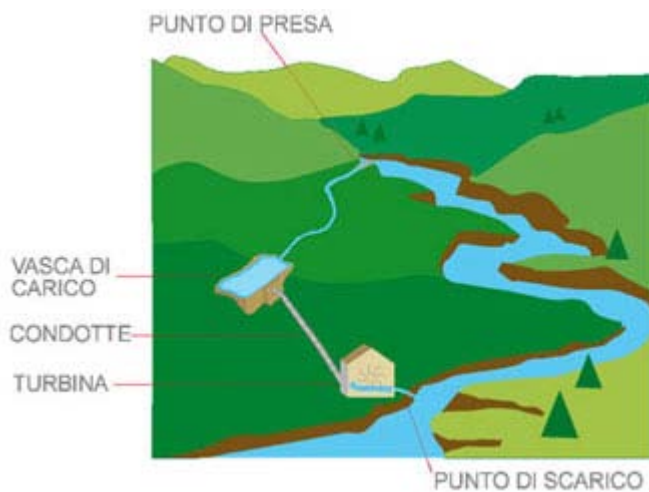
Fig 38. Funzionamento di un impianto di micro-idro ad acqua fluente ( http://www.casasoleil.it )
