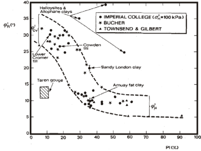
Fig. 7.5 – Angolo di attrito efficace in funzione dell'indice di plasticità (PI) per terreni coesivi (Lupini et al., 1981).
