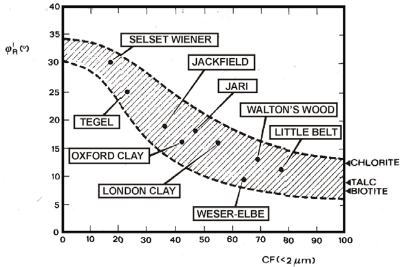
Fig. 7.6 – Angolo di attrito efficace in funzione del contenuto di argilla (CF) per terreni coesivi (Skempton, 1964).
