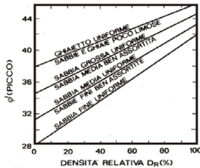
Fig. 7.1 – (angolo d'attrito di picco in termini di sforzi efficaci) in funzione della densità relativa ( D_R ) per differenti terreni non coesivi (SCHMERTMANN, 1978).
