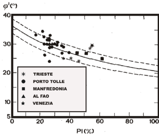
Fig. 7.4 – Valori indicativi dell'angolo \phi' funzione dell'indice di plasticità (PI) per terreni coesivi normal consolidati (Jamiolkowski et al., 1979).
