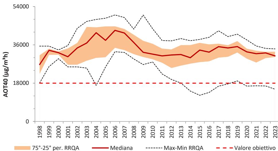
Figura 1.28: trend AOT40 medio su 5 anni
