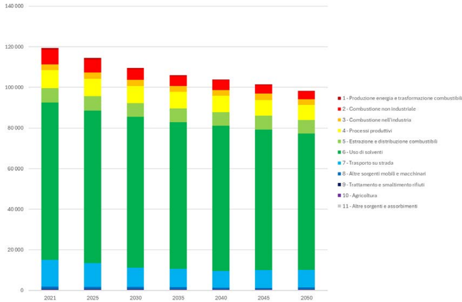
Figura 3.1.a. Proiezione delle emissioni in Lombardia di COV (non biogenici) tra il 2021 ed il 2050 (Elab. ARPA Lombardia).
