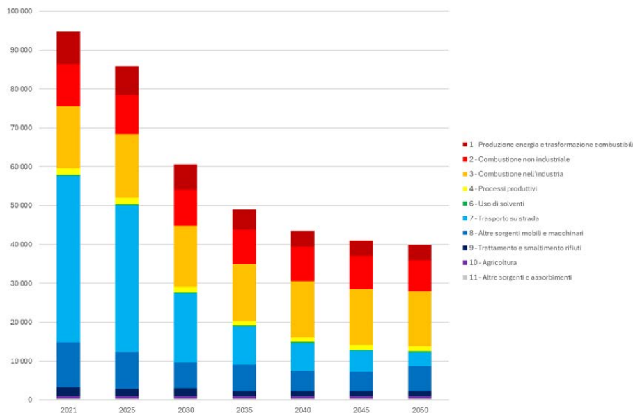
Figura 3.1.b. Proiezione delle emissioni in Lombardia di NO x tra il 2021 ed il 2050 (Elab. ARPA Lombardia).
