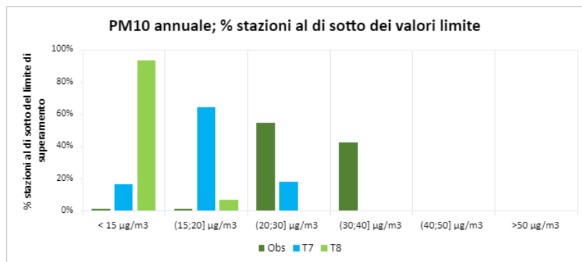
Figura 3.3. a) Applicazione del modello NINFA-ER alle stazioni del bacino padano e b) Applicazione del modello SMAL-LO alle stazioni della Regione Lombardia
