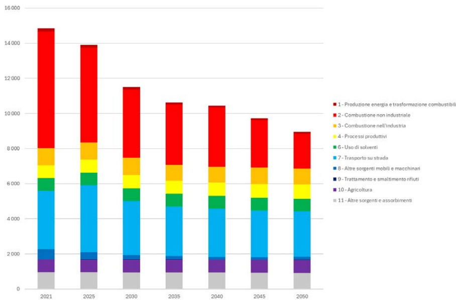
Figura 3.1.d. Proiezione delle emissioni in Lombardia di PM 10 tra il 2021 ed il 2050 (Elab. ARPA Lombardia).
