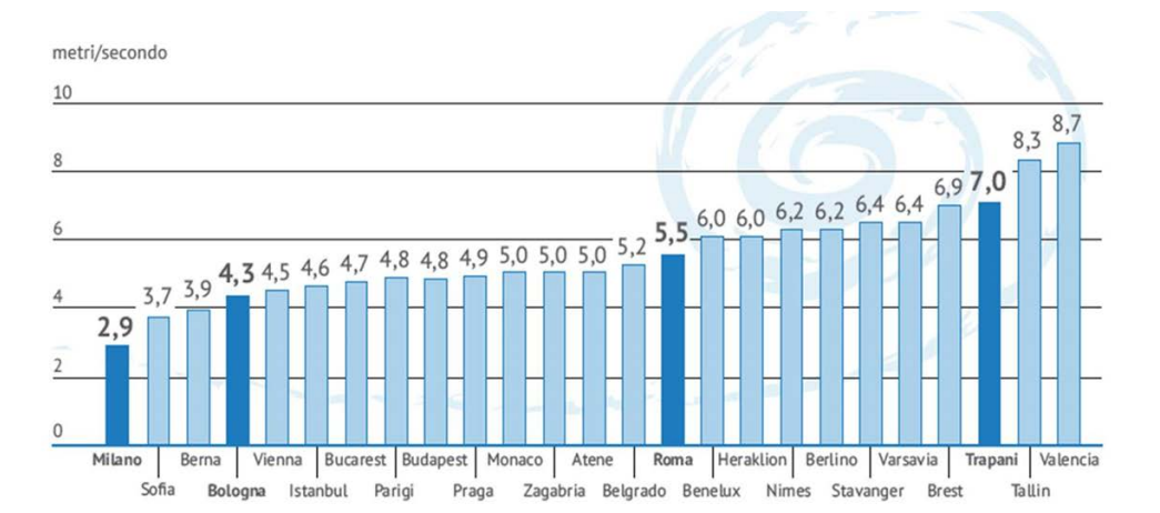
Figura 1.1. Life Prepair, elaborazioni da WMO anno 2016 -2017
