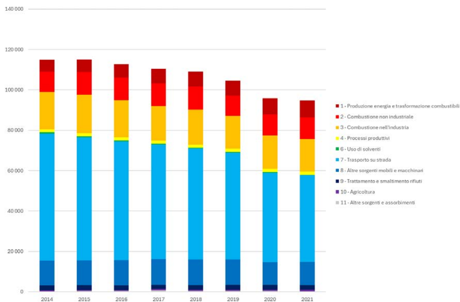
Figura 2.3.b. Emissioni in Lombardia di NO x tra il 2014 ed il 2021 (Elab. ARPA Lombardia).
