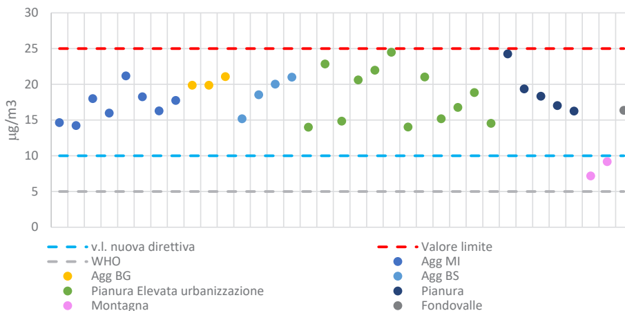
Figura 1.4. PM2.5- Media annua per stazione
