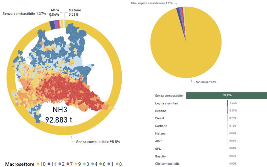
Figura 2.2.d. Emissioni in Lombardia di NH 3 nel 2021 (Fonte: ELABORAZIONI ARPA LOMBARDIA) 4 .
