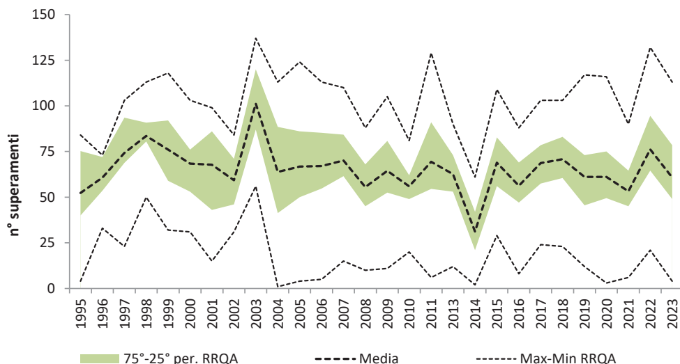
Figura 1.23. Andamento del numero di superamenti annuali dell'obiettivo a lungo termine per l'O3
