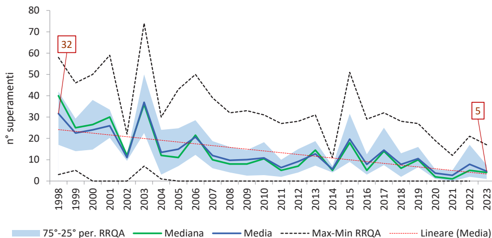
Figura 1.25: Andamento del n° di giorni di superamento della soglia di informazione (180 mg/m³)
