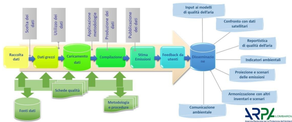
Figura 2.1 schema delle principali attività che compongono la redazione di un inventario di emissioni in atmosfera
