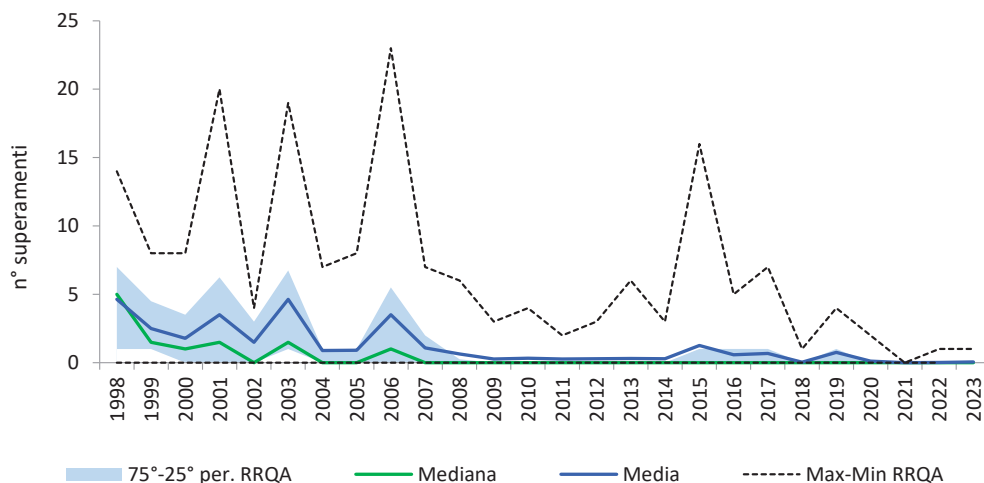
Figura 1.26: Andamento del n° di giorni di superamento della soglia di allarme (240 mg/m³)
