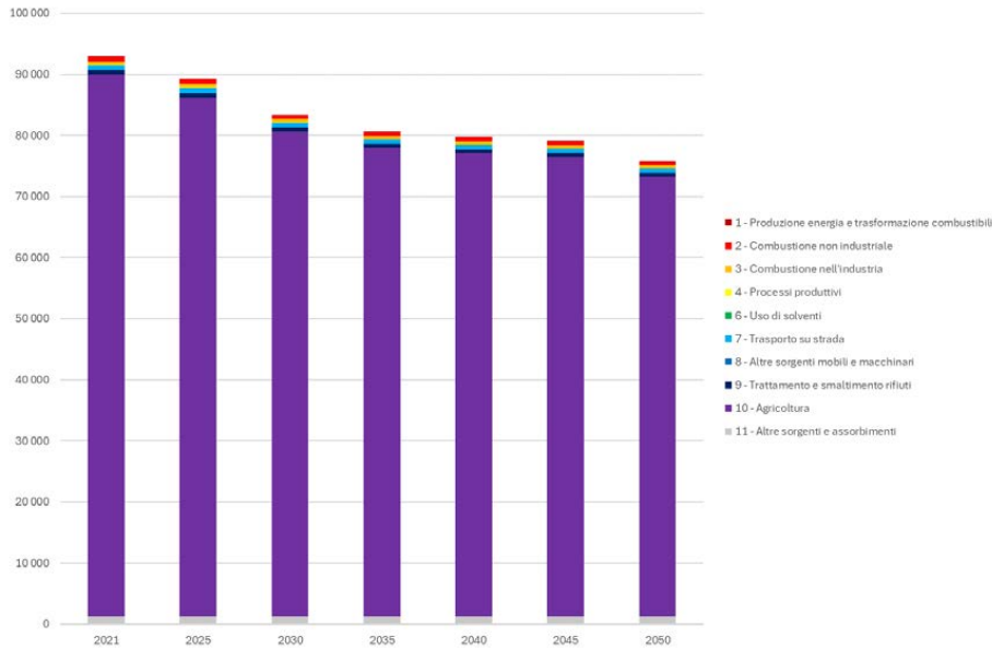
Figura 3.1.c. Proiezione delle emissioni in Lombardia di NH 3 tra il 2021 ed il 2050 (Elab. ARPA Lombardia).
