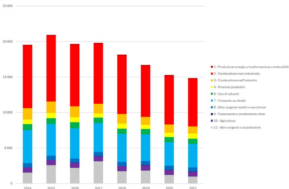
Figura 2.3.d. Emissioni in Lombardia di PM 10 tra il 2014 ed il 2021 (Elab. ARPA Lombardia).
